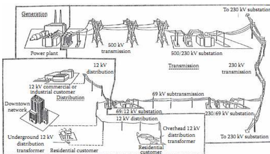
Рис. 12: Концепция передачи электроэнергии
